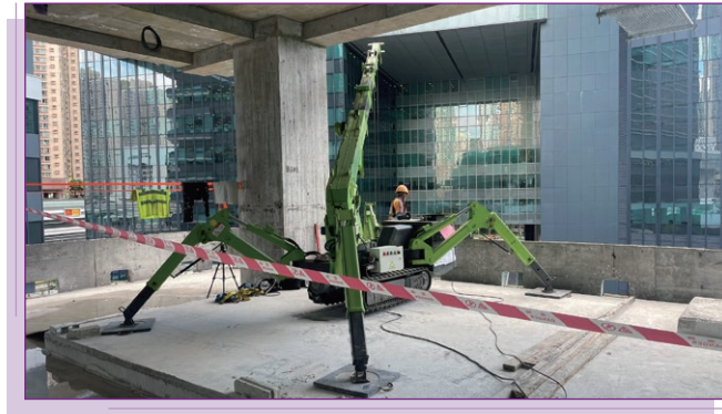
Spider crane 蜘蛛式起重機
