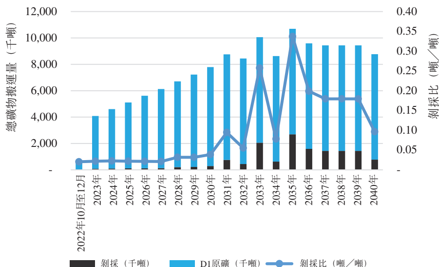
圖6-8：採礦年限內的生產計劃
